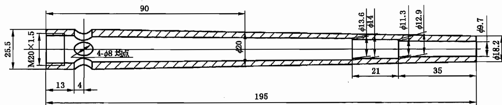
a) 喷嘴
