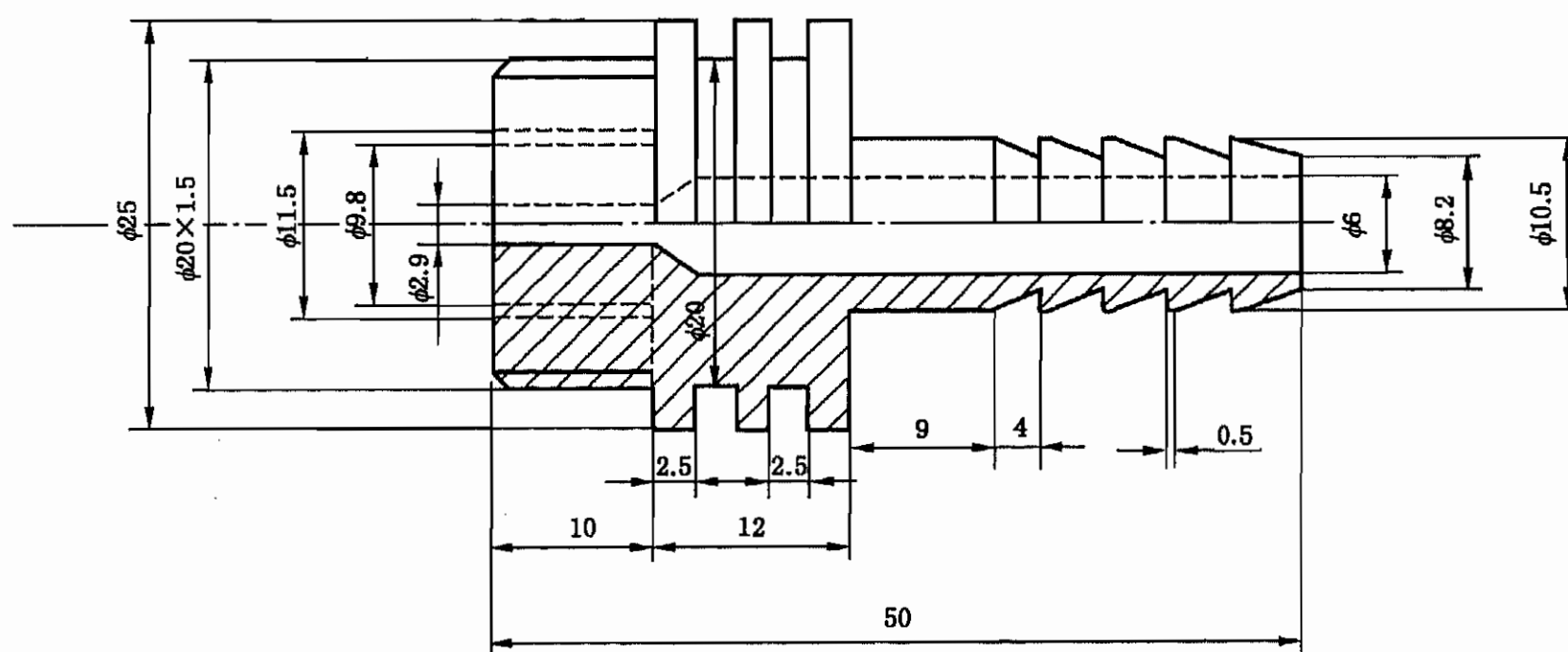
b) 喷嘴芯
