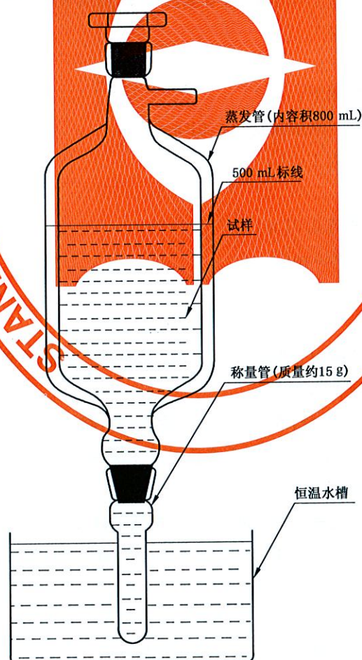
图 1 蒸发器
