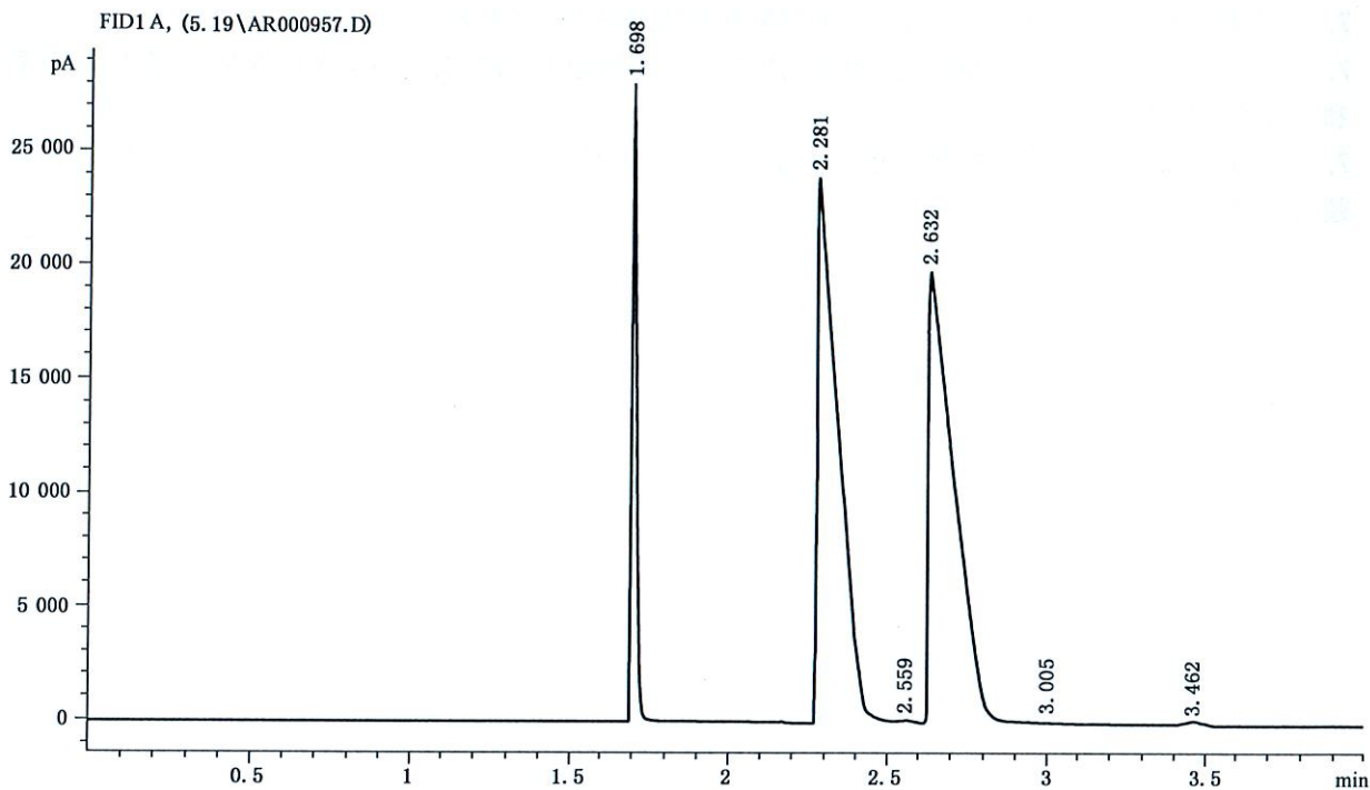
图 A.1 六氟丙烷两种同分异构体色谱图例
