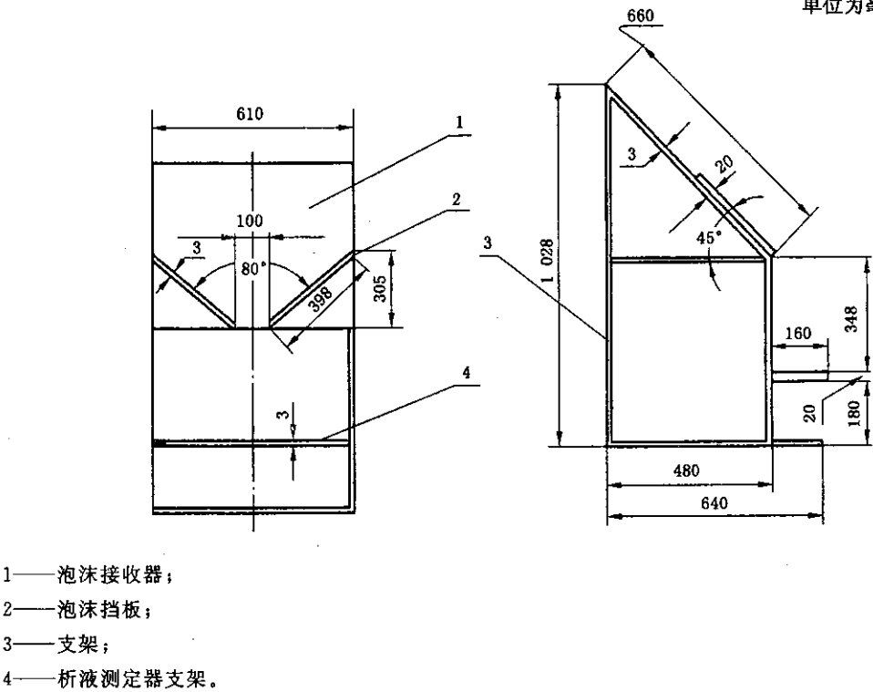
图 4 低倍泡沫收集器示意图
