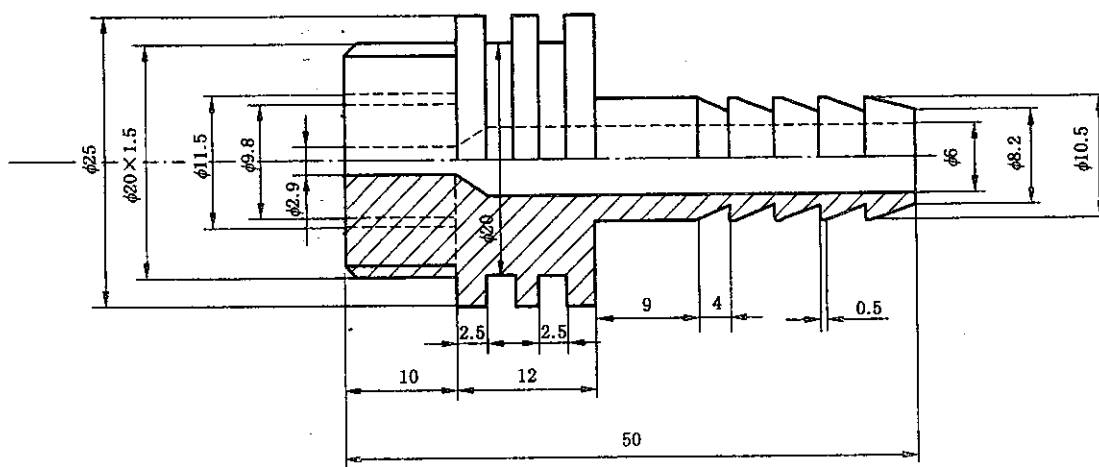
b) 喷嘴芯
