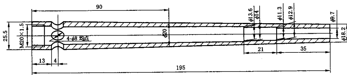
a) 喷嘴
