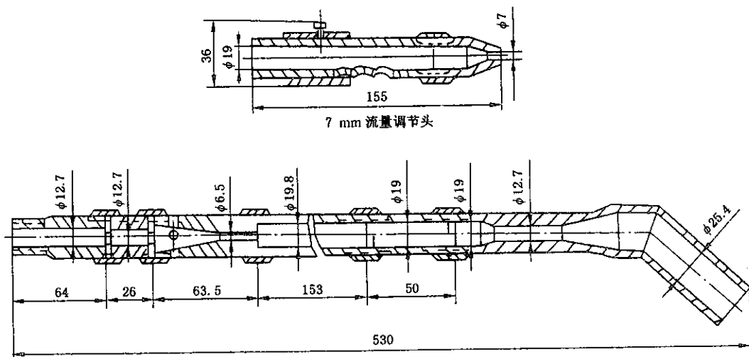
图 A.1 5 L/min 泡沫枪及附件
