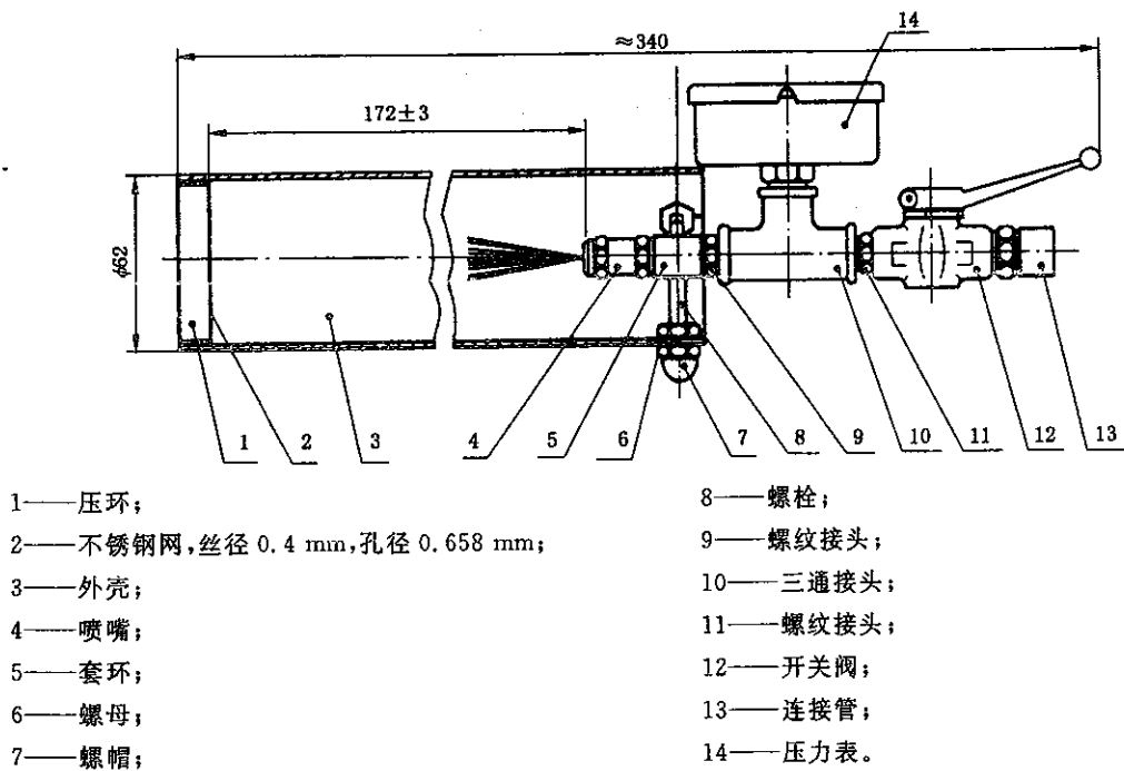
图 7 中倍泡沫产生器
