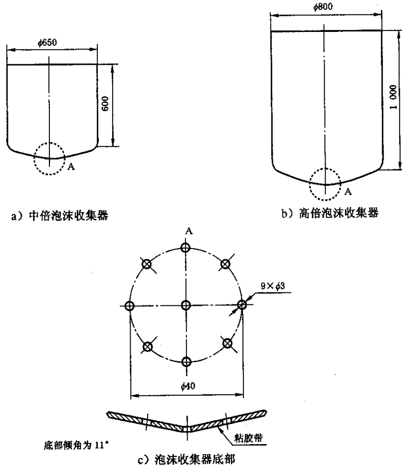
图 6 泡沫收集器
