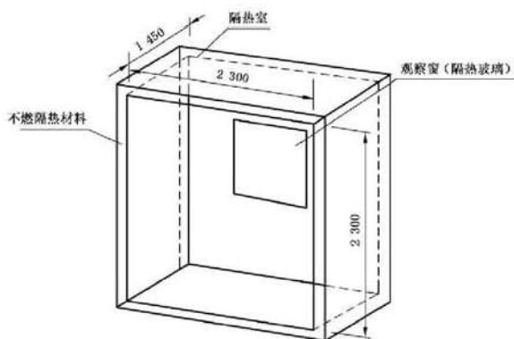
图 1 隔热室
