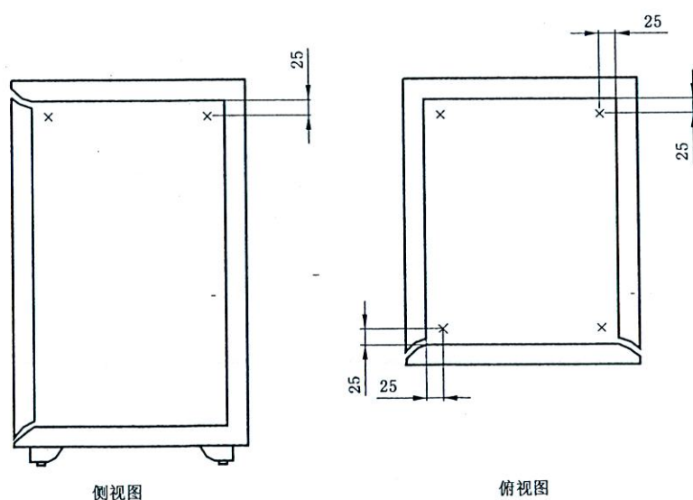
图4 D类和DIS类单扇门试件内部测温点布置示意图
