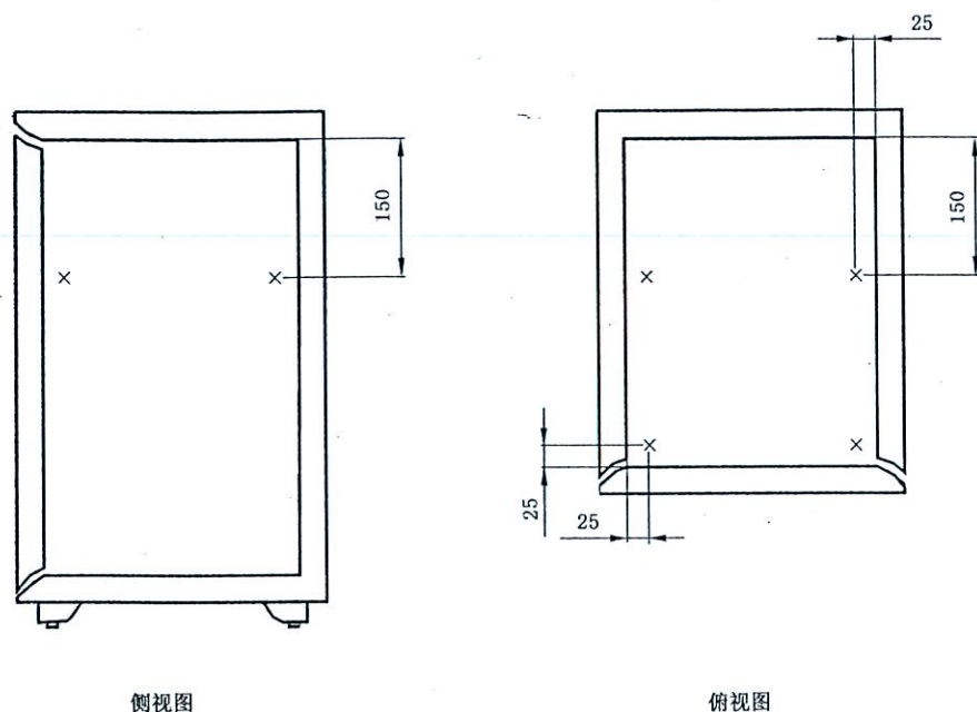
图1 P类单扇门试件内部测温点布置示意图
