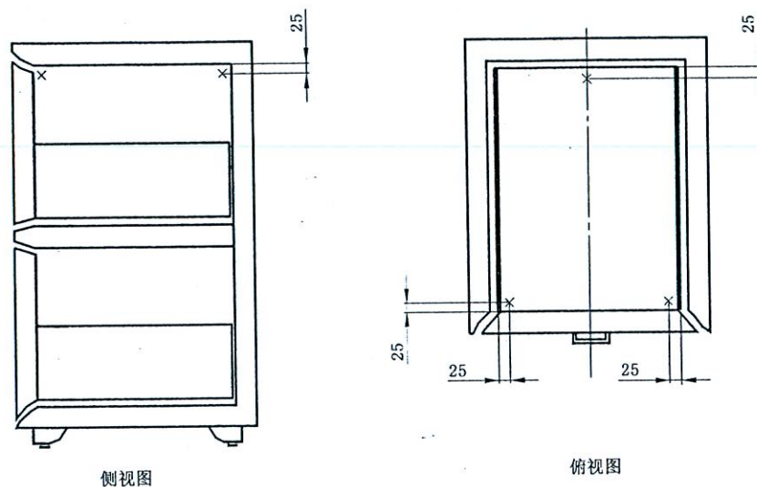
图 5 D 类和 DIS 类试件第 1 层抽屉测温点布置示意图
