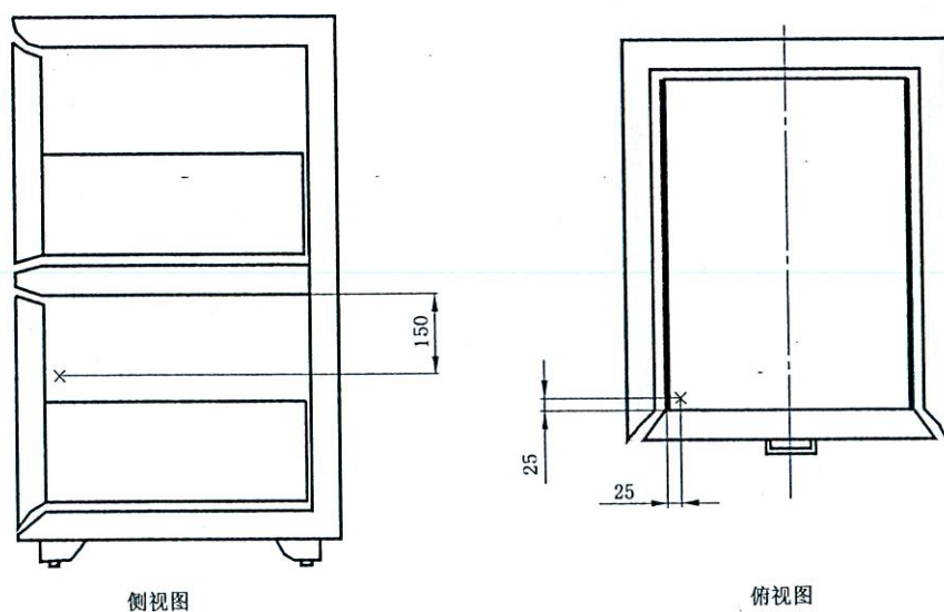
图3 P类试件第2层抽屉测温点布置示意图
