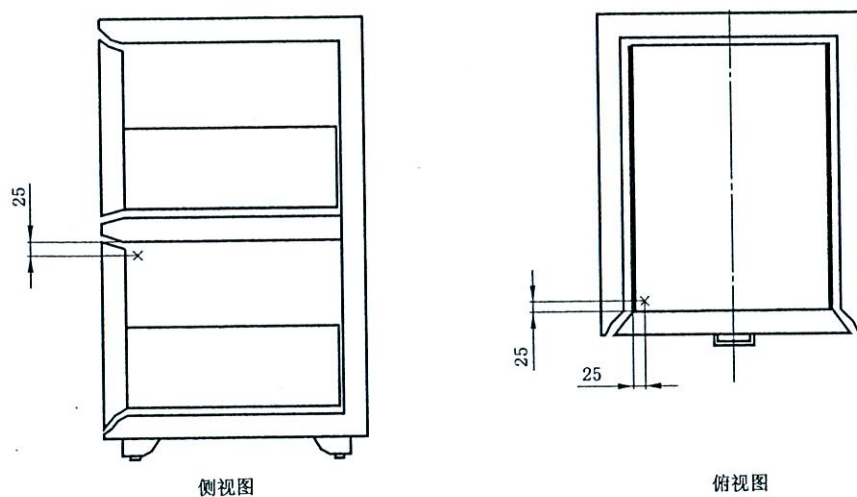
图 6 D 类和 DIS 类试件第 2 层抽屉测温点布置示意图
