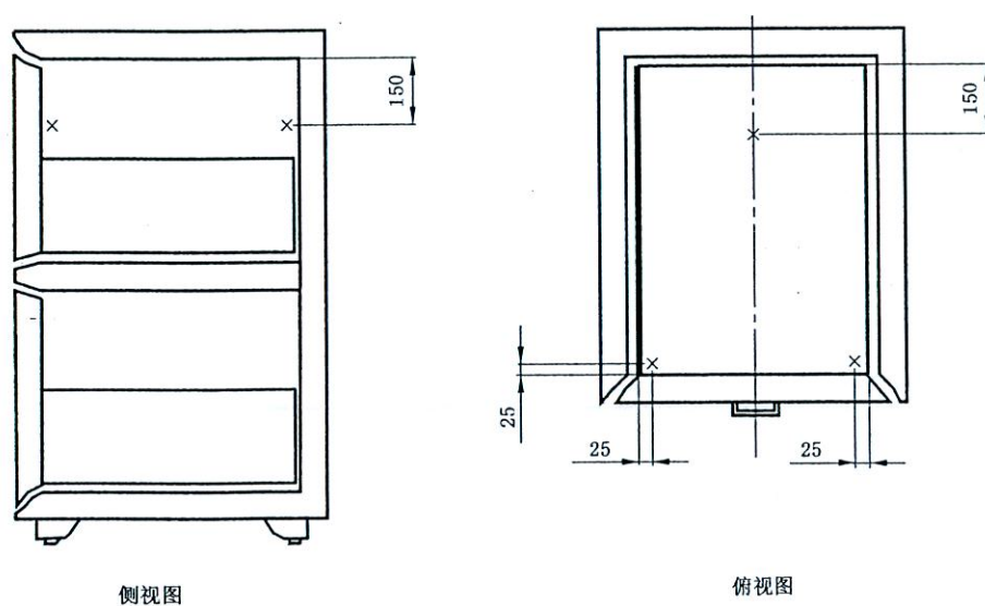
图2 P类试件第1层抽屉测温点布置示意图
