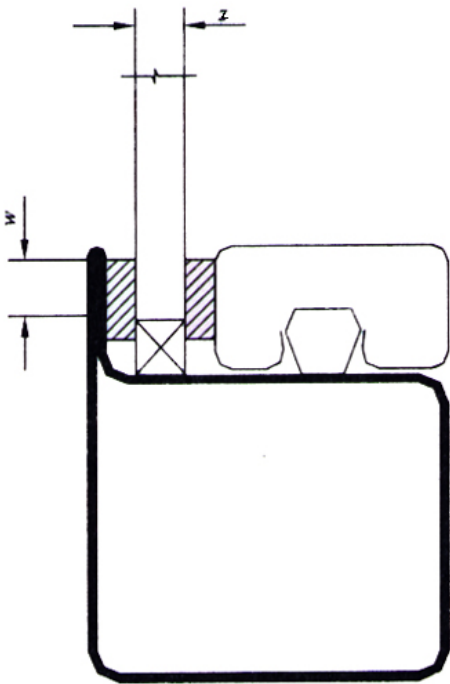
图 1 镶玻璃构件立面示意图
