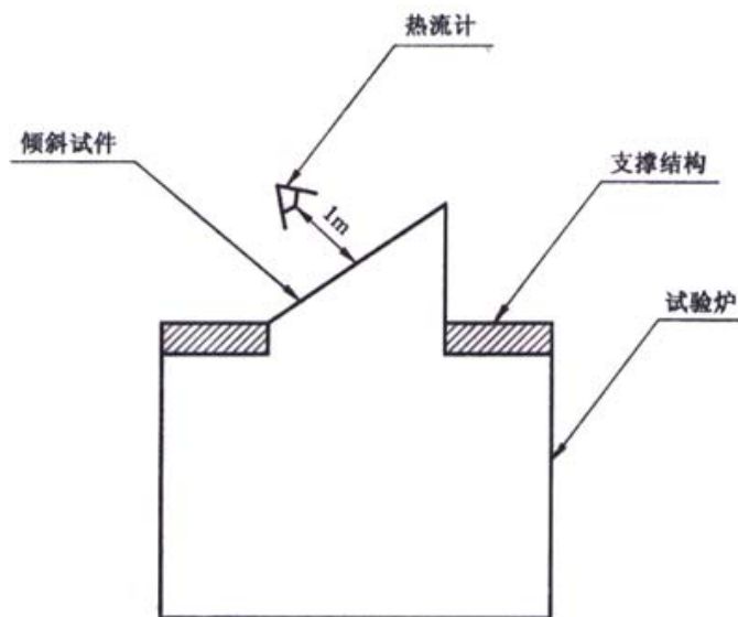
图 5 倾斜镶玻璃试件热流计的测量位置
