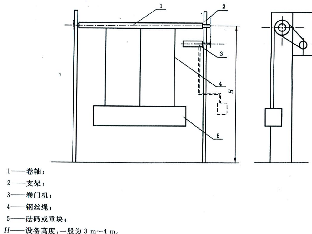
图 A.1 基本性能试验设备示意图
