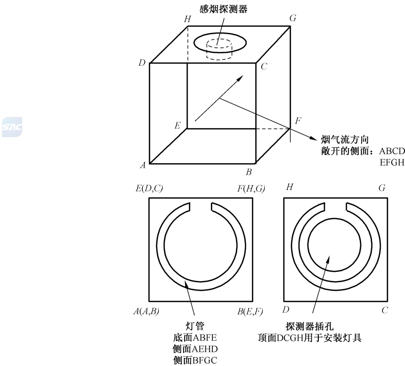
图 D.1 闪光装置图
