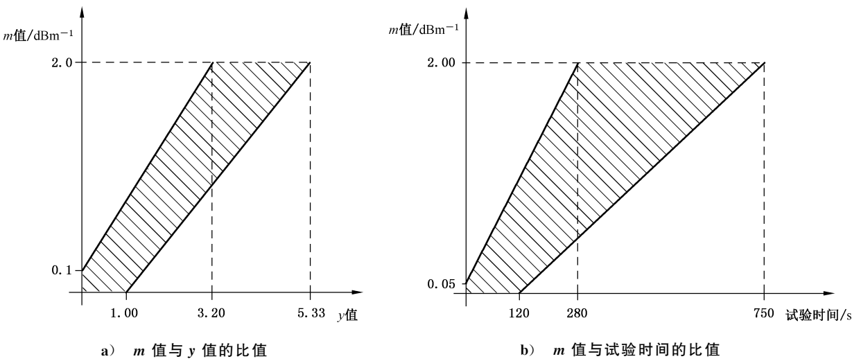
图 G.2 试验火合格判据
