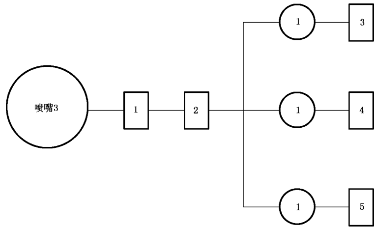
图 B. 2 喷嘴试验程序图
