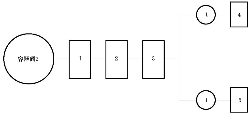
图 B. 1 容器阀试验程序图
