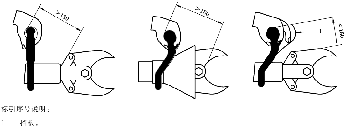
图 1 把手防护要求示意图
