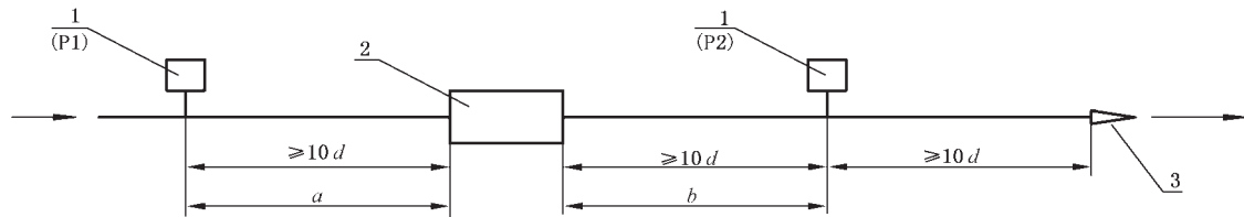
c) 容器阀压力损失测试装置
