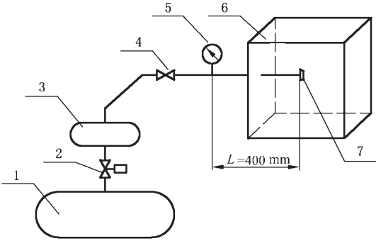
b) 悬挂方式 图 3 (续)
