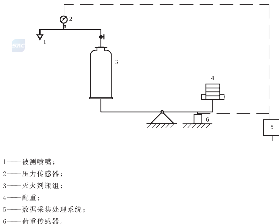
a) 质量平衡方式
