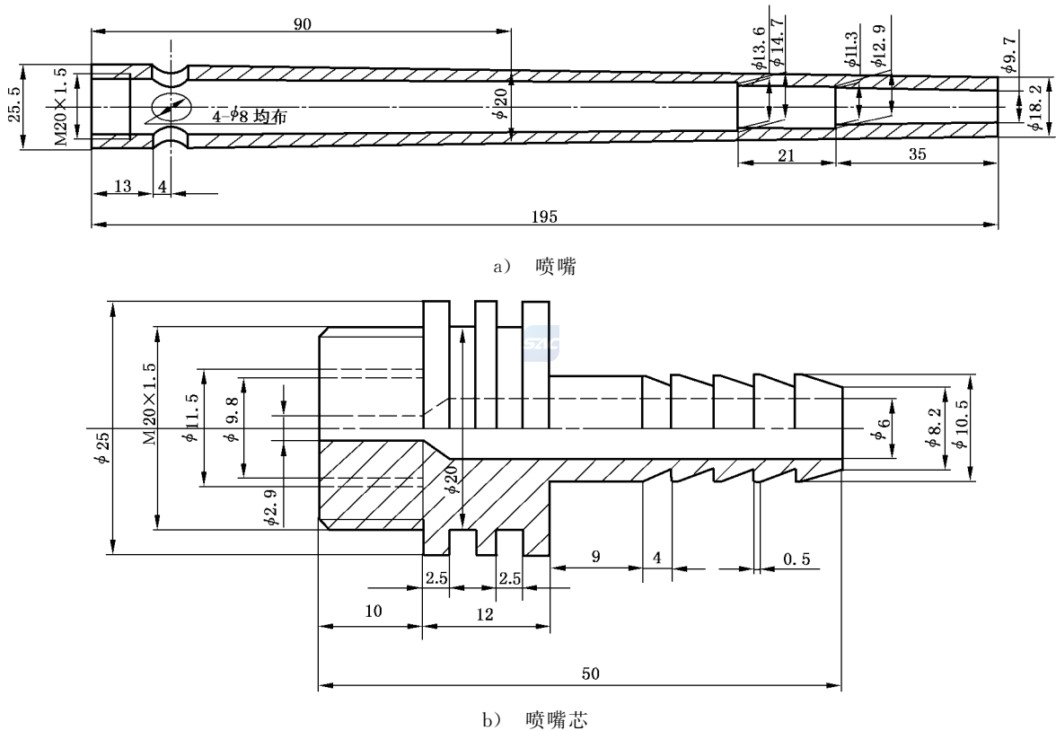
图 1 喷嘴
