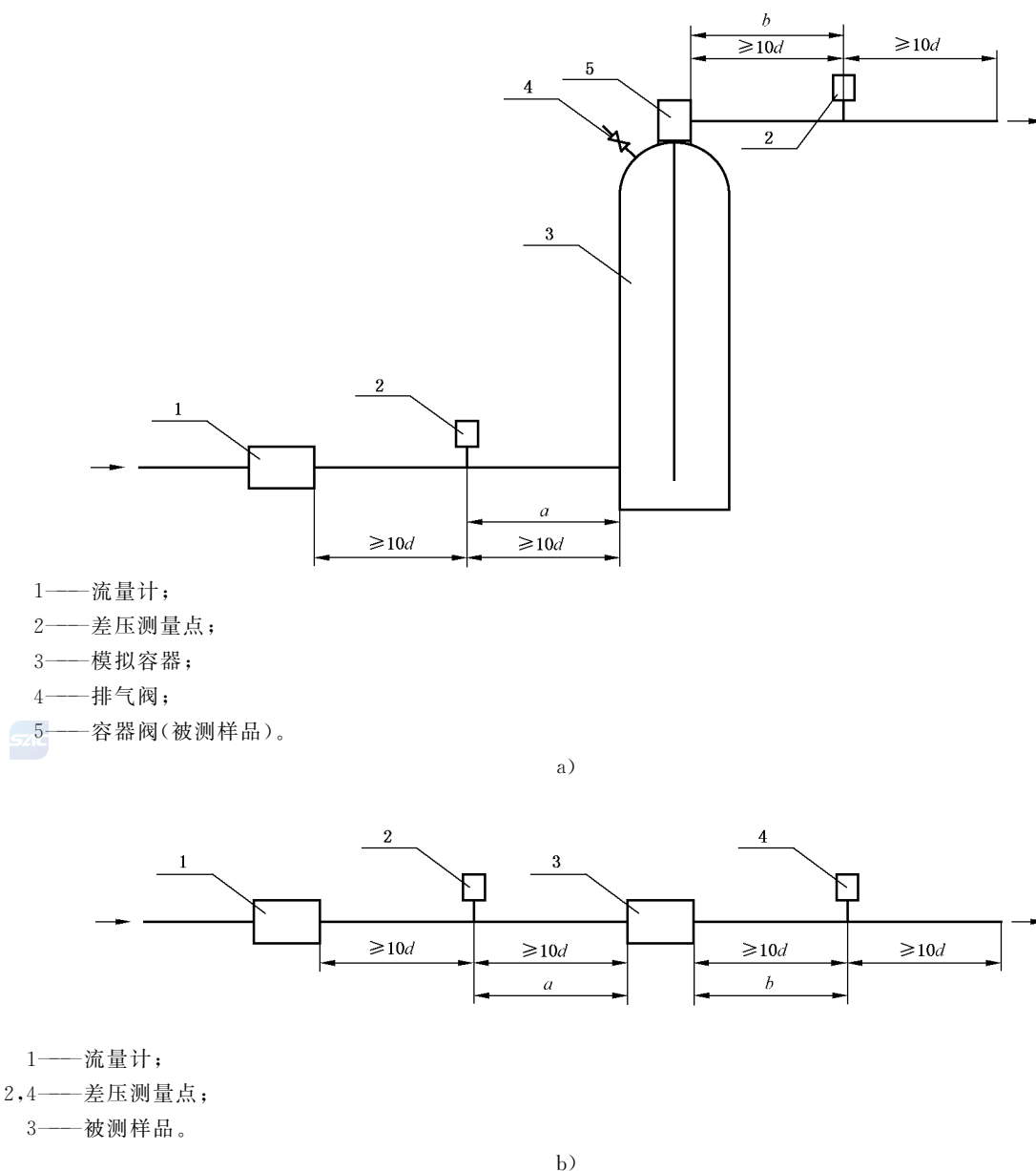
图 1 等效长度试验装置
