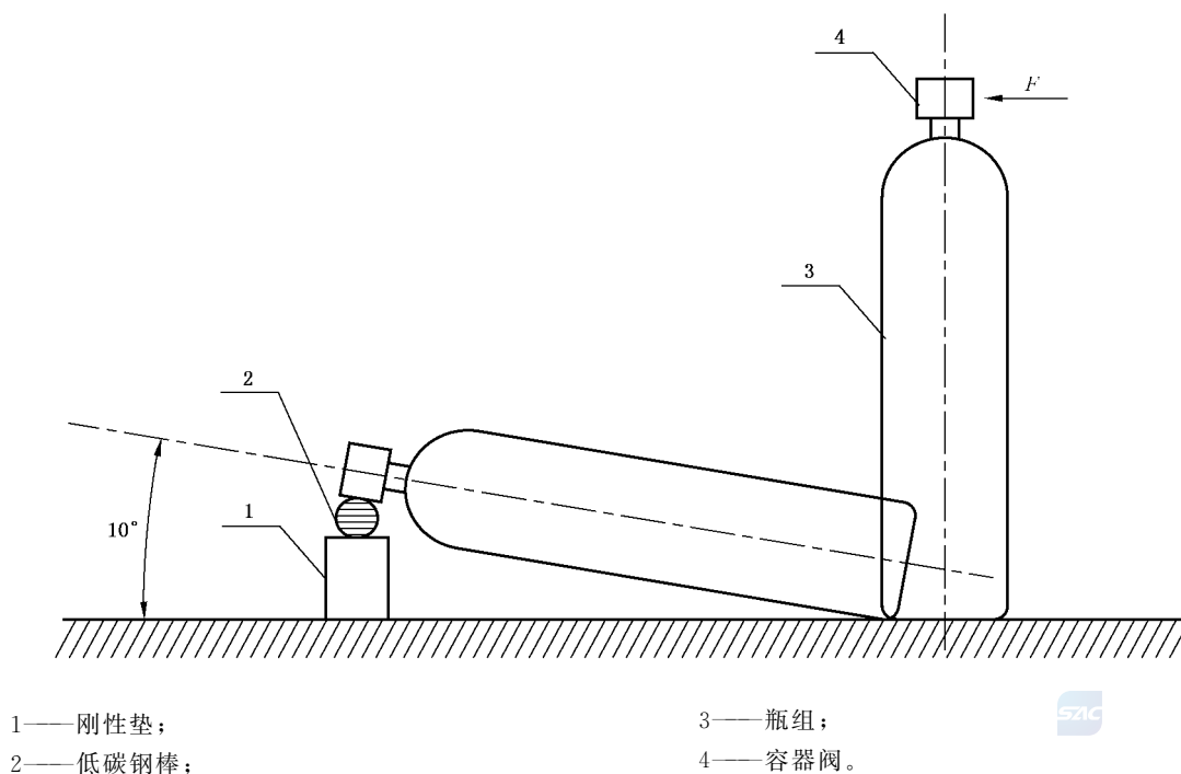
图 2 倾倒冲击试验示意图
