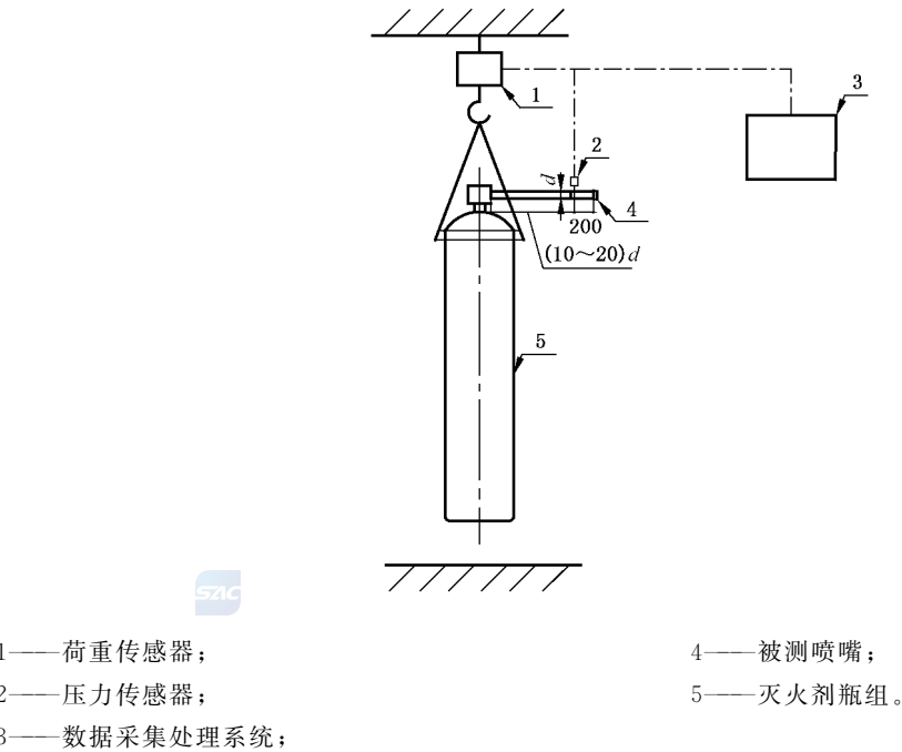
b) 悬挂方式
