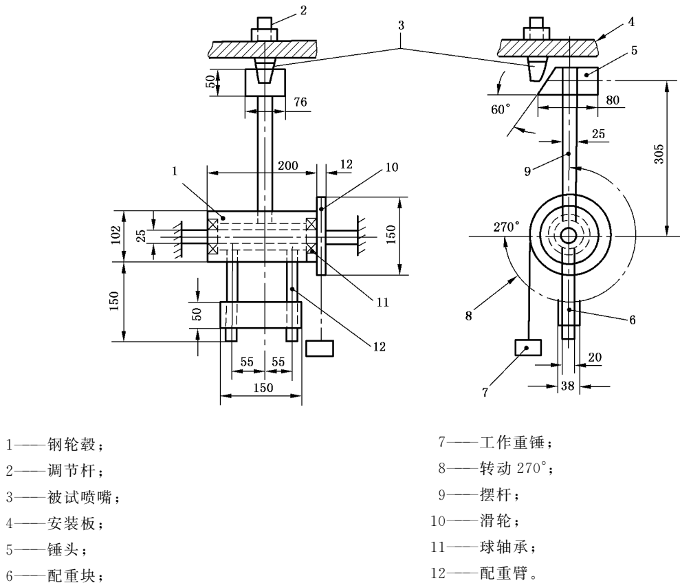
图 10 喷嘴耐冲击试验装置
