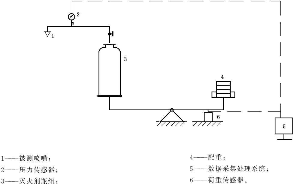
a) 重量平衡方式
