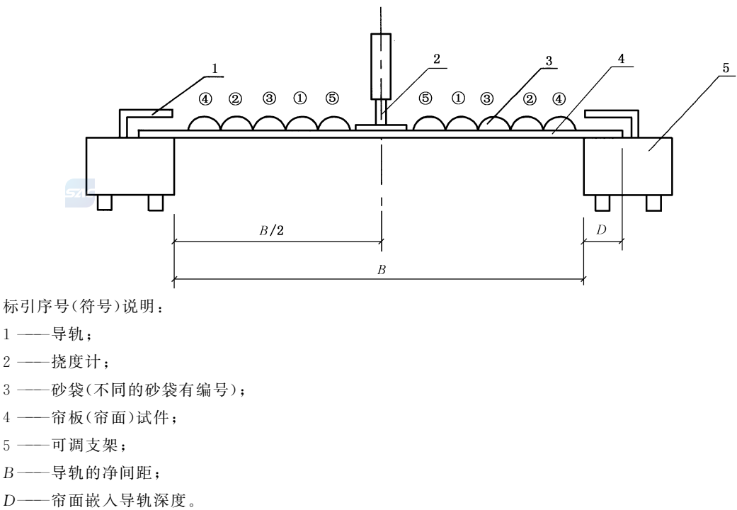
图 9 耐风压性能试验设备示意图
