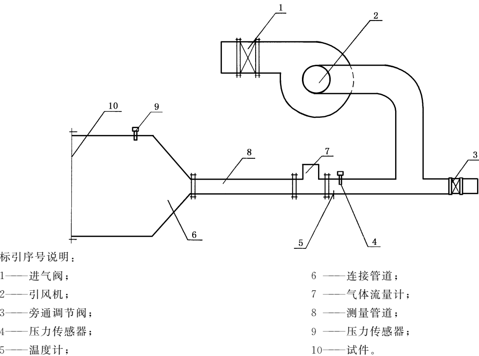
图 10 帘面漏烟量试验设备示意图
