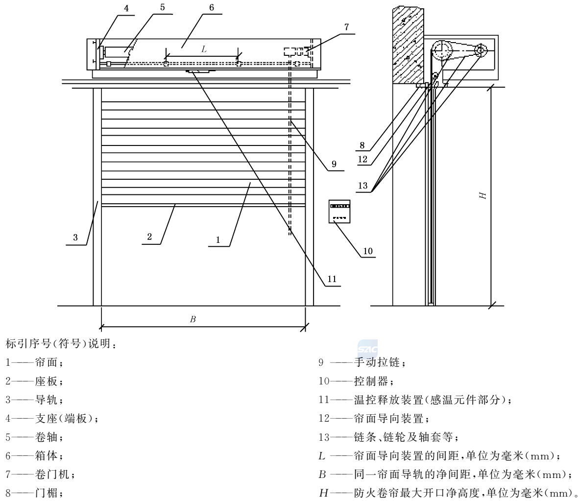
图 1 防火卷帘组成结构示意图
