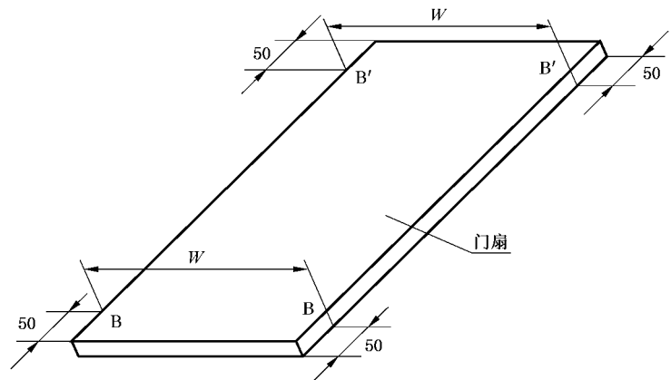
图 2 门扇宽度测量位置示意图
