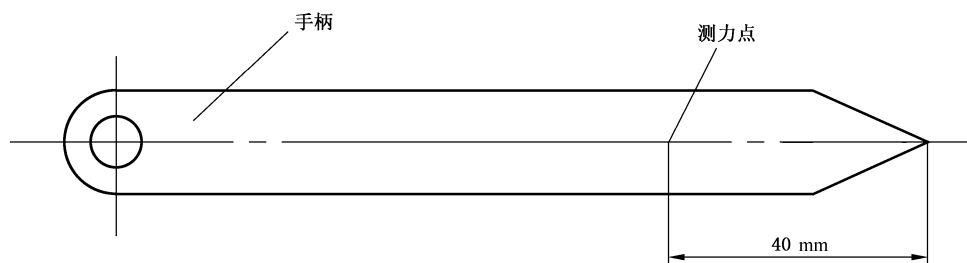
图 4 启闭力测力位置
