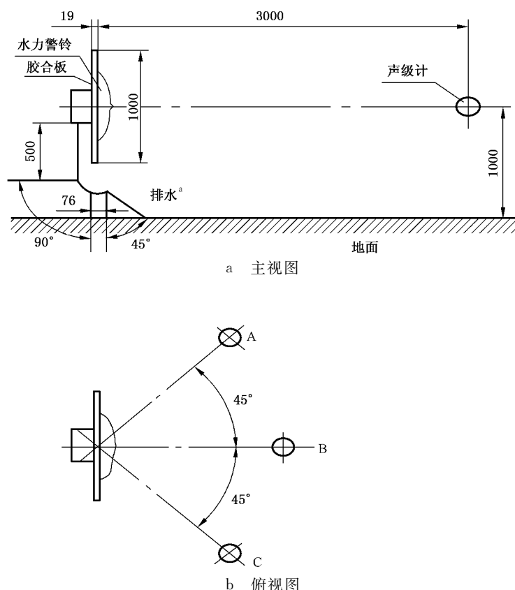
图 3 响度试验的试验布置
