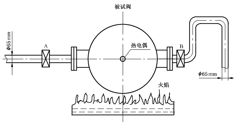
图 4 耐火试验的试验布置
