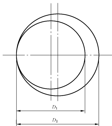
图 1 直径方向间隙 = D_2 - D_1
