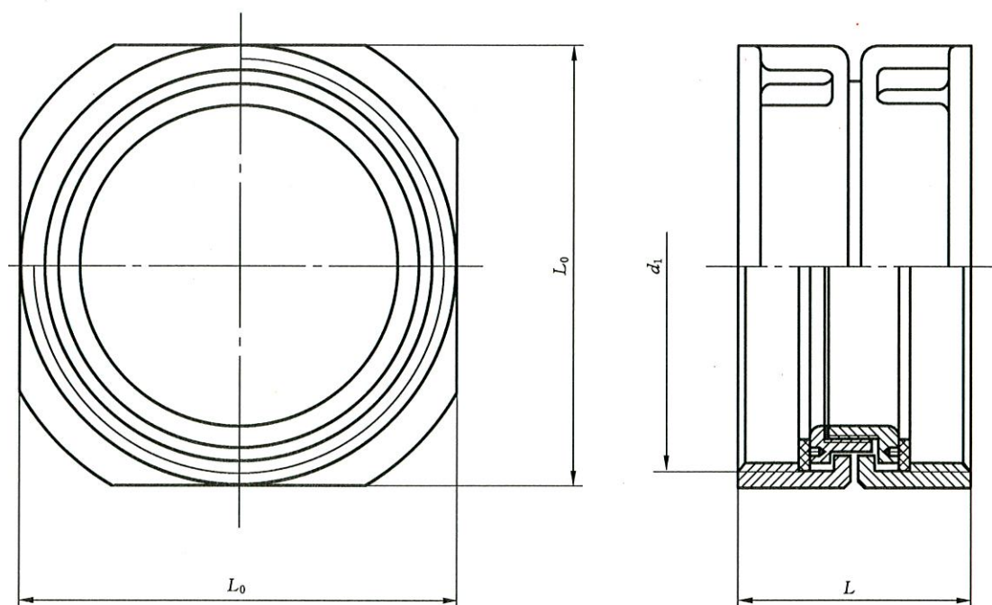
图 3 KT 型同型接口
